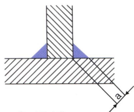
L角焊縫
